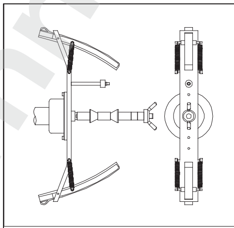
Рис. 4.3 Установка образцового грузика на внешней стороне фланца для МОТО-колес на валу (фаза Cal3)
